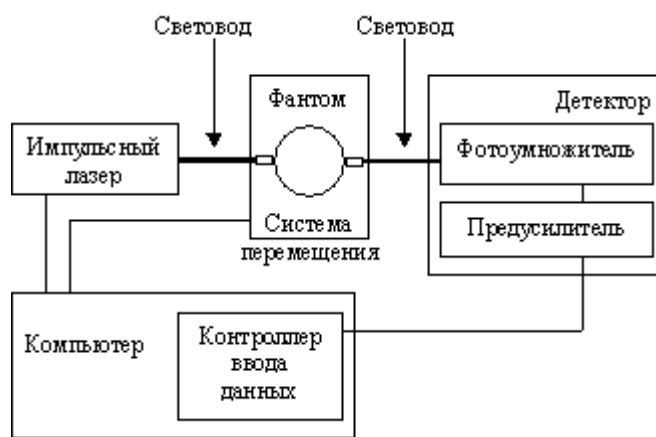
Рисунок 3.2 – Схема трансмиссионного оптического томографа
